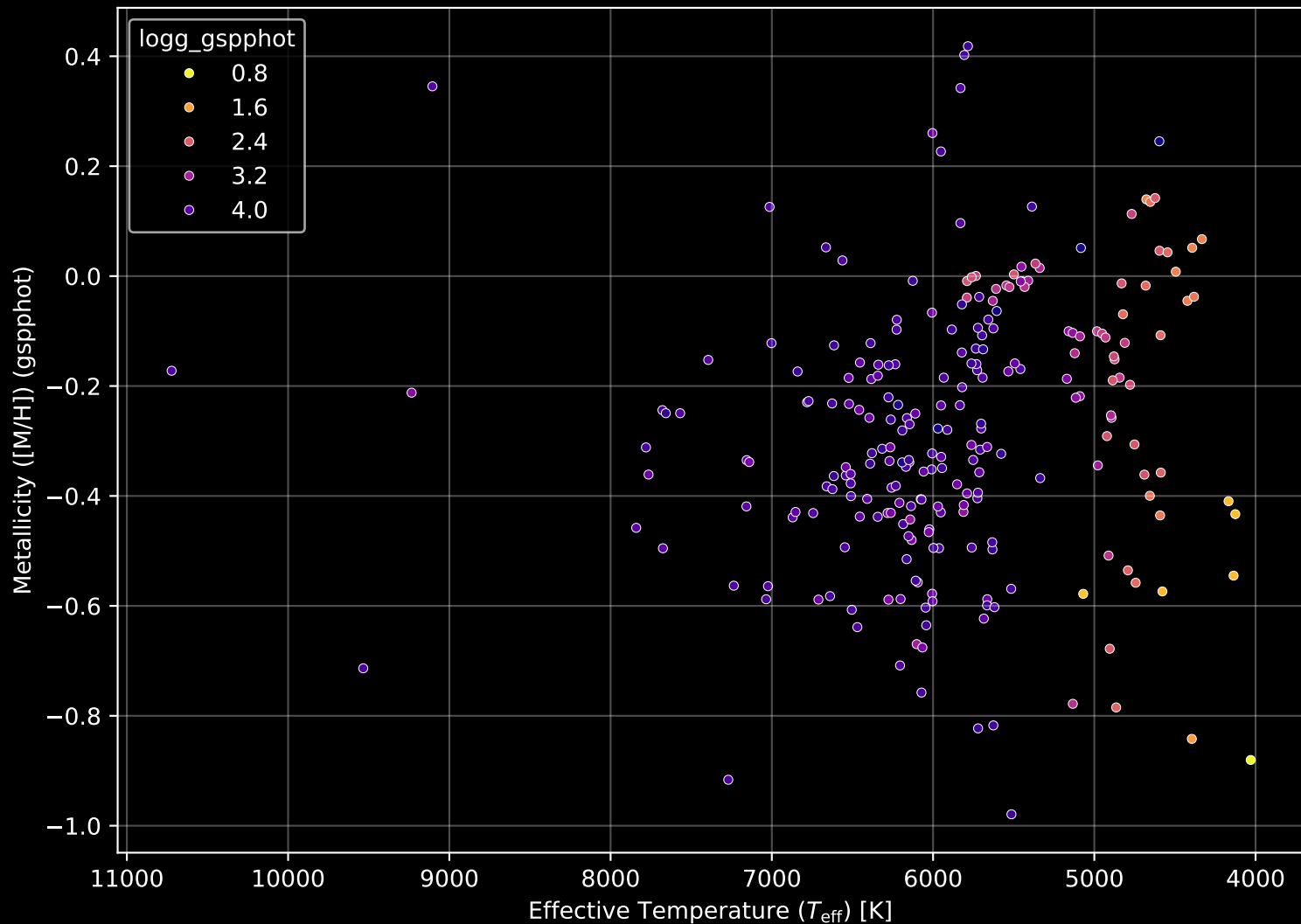
GALAH DR4 Field: [8290] Stellar Population Parameters (n= 242)
