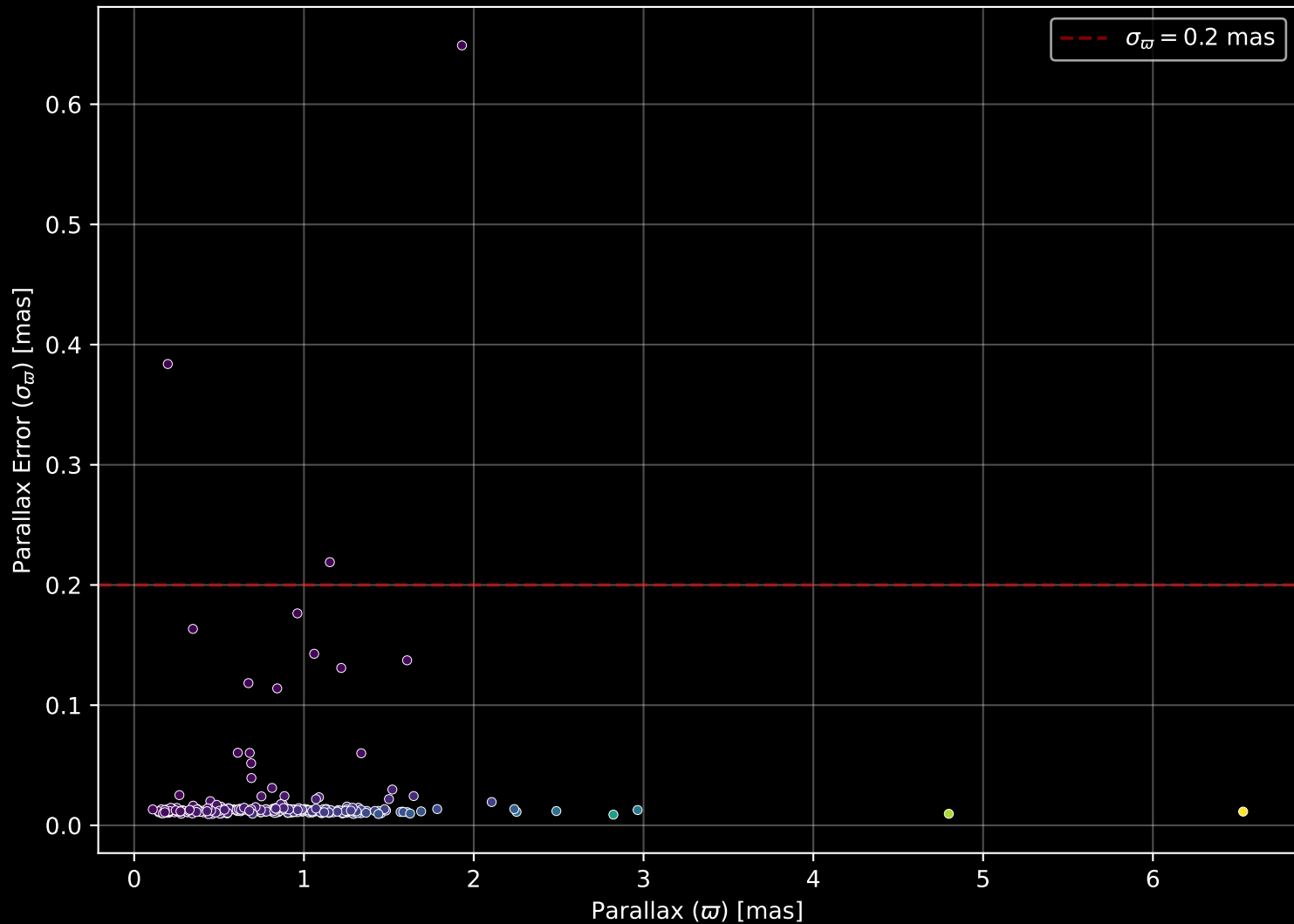
GALAH DR4 Field: [8290] Parallax Quality (n= 242)
