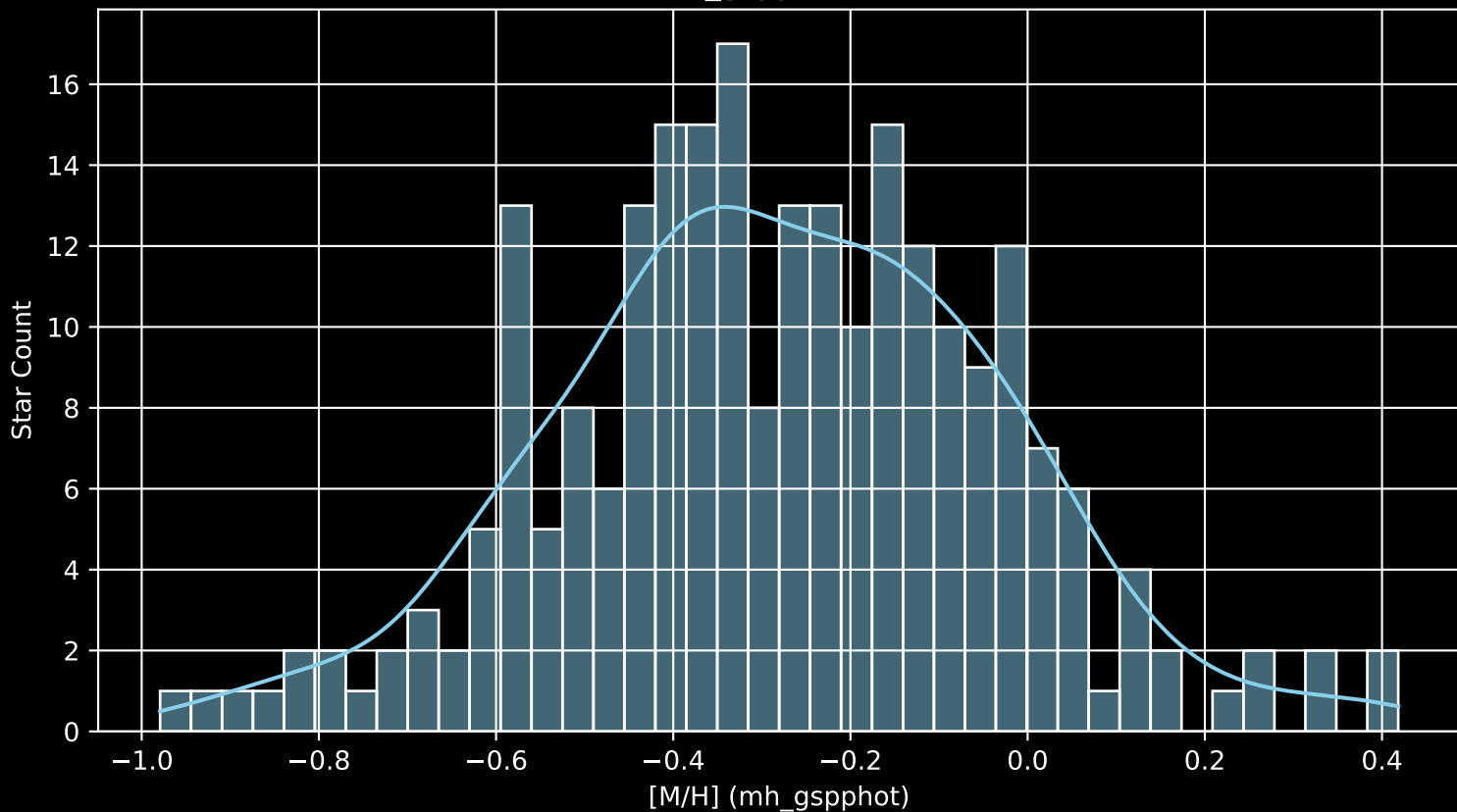
GALAH DR4 Field: [8290] [M/H] (mh_gspphot) (n= 242)
